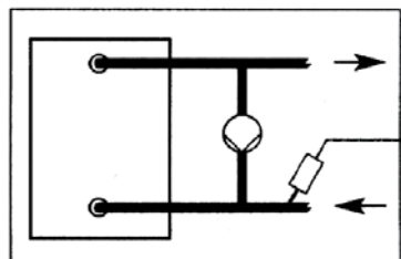
Датчик теплоносителя на возврате в котел
